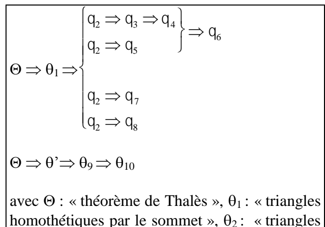
Figure 6 – Schéma d'une organisation mathématique régionale autour du théorème de Thalès
