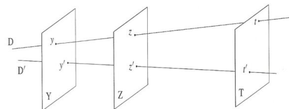
Figure 3 – La figure accompagnant le théorème de Thalès
