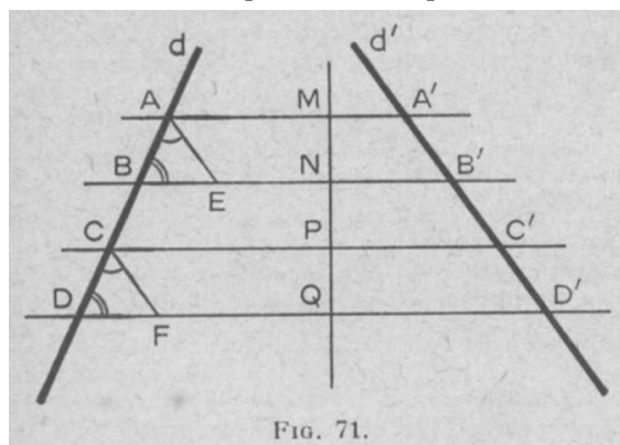
Figure 5 – La figure accompagnant le théorème des parallèles équidistantes
