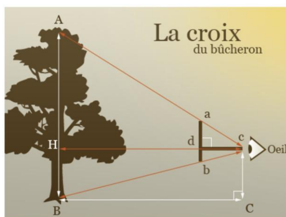
Figure 7 – Schéma représentant l'estimation de la hauteur d'un arbre à l'aide de la croix du bûcheron
