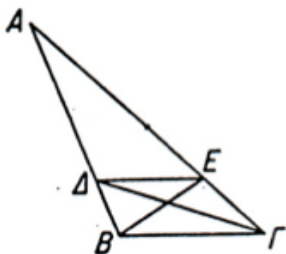
Figure 1 – La figure accompagnant la proposition 2 du livre VI
