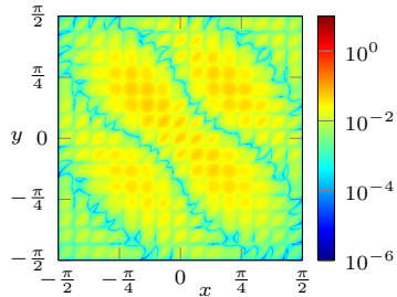
Absolute FEM error |u - u_h|
