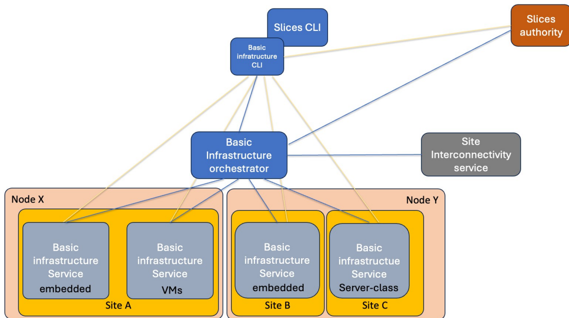
Figure 1: Architecture distribuée SLICES-RI
