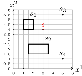
Fig. 4: Localisation uncertainty
