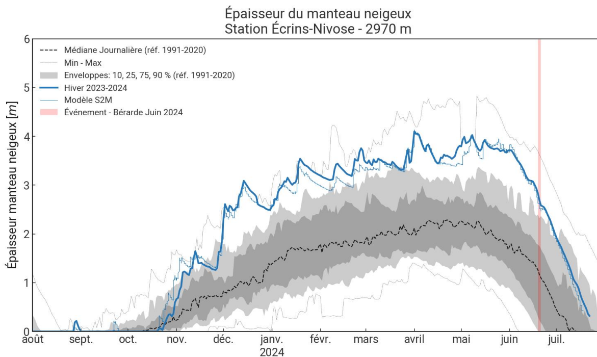
Figure 52: Épaisseur du manteau neigeux à la station nivôse des Ecrins (44.94N, 6.35E) pour l'hiver 2023-2024 (trait bleu) en rapport à la climatologie des observations de 1991 à 2020. Source : CNRM/CEN.
