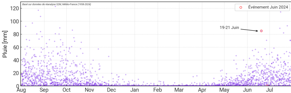
Figure 49: Saisonnalité des lames d'eau de pluie sur 48h sur le bassin versant des Etançons sur la période 1958-2024. L'épisode du 19 juin 7h au 21 juin 7h est mis en évidence. Source : CNRM/CEN.
