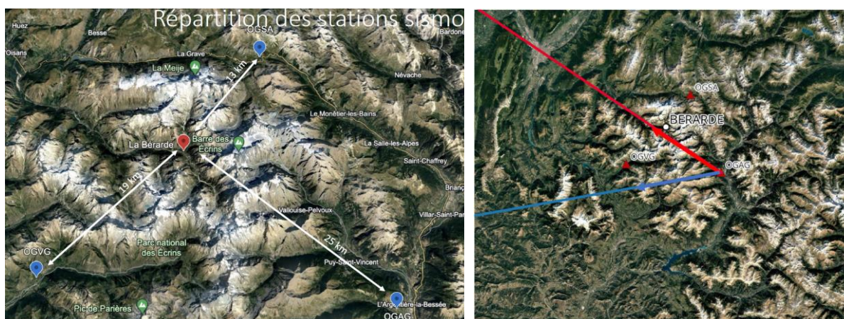
Figure 31: Gauche : emplacement des sismographes dans les Ecrins. Droite : changement de la direction d'origine du bruit sismique de la station d'Argentière le 21 juin.
