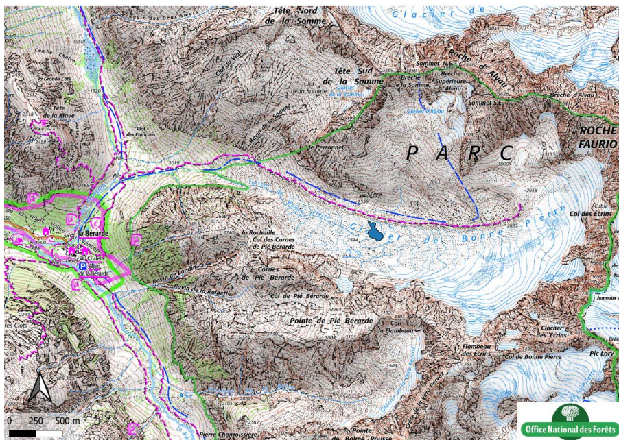
Figure 65: Emplacement du lac supraglaciaire, en bleu
