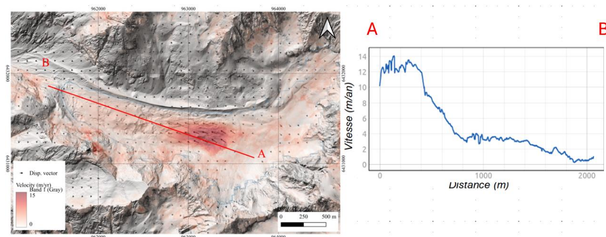
Figure 61: Carte de vitesse d'écoulement du glacier de Bonne Pierre moyennée sur la période 2003-2024 établie à partir des images aériennes et satellites à haute résolution (1 m). Profil de vitesse obtenu le long de la ligne longitudinale d'écoulement A-B. Source : ISTerre.
