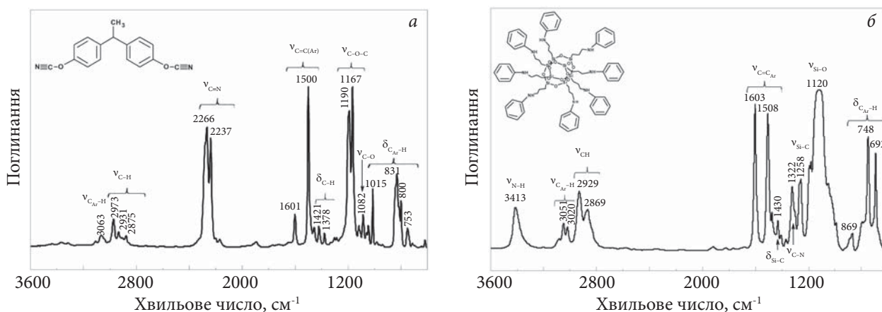
Рис. 4. ФТІЧ спектри (в області 3600–600 \text{cm}^{-1} ) індивідуальних (а) ДЦБЕ і (б) NPAP-POSS
