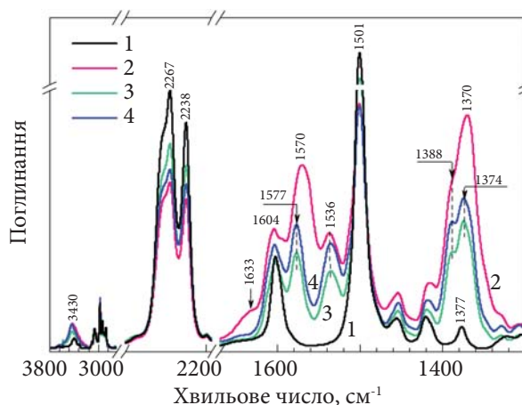
Рис. 3. ФТГЧ спектри (в діапазоні 3800–1300 \text{cm}^{-1} ) сумішей ДЦБЕ/NPAP-POSS (90/10 мас.%) після диспергування наноаповнювача різними методами: 1 – вихідна суміш ДЦБЕ/NPAP-POSS; 2 – ДЦБЕ/NPAP-POSS M3(165) ; 3 – ДЦБЕ/NPAP-POSS M3(65) ; 4 – ДЦБЕ/NPAP-POSS У3(65)
