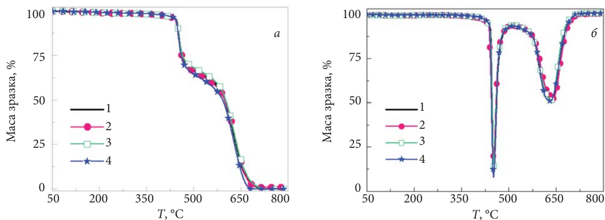
Рис. 7. Криві (а) ТГА і (б) ДТГ для зразків: 1 – ПЦС; 2 – ПЦС/NPAP-POSS M3(165) ; 3 – ПЦС/NPAP-POSS M3(65) ; 4 – ПЦС/NPAP-POSS УЗ(65)
