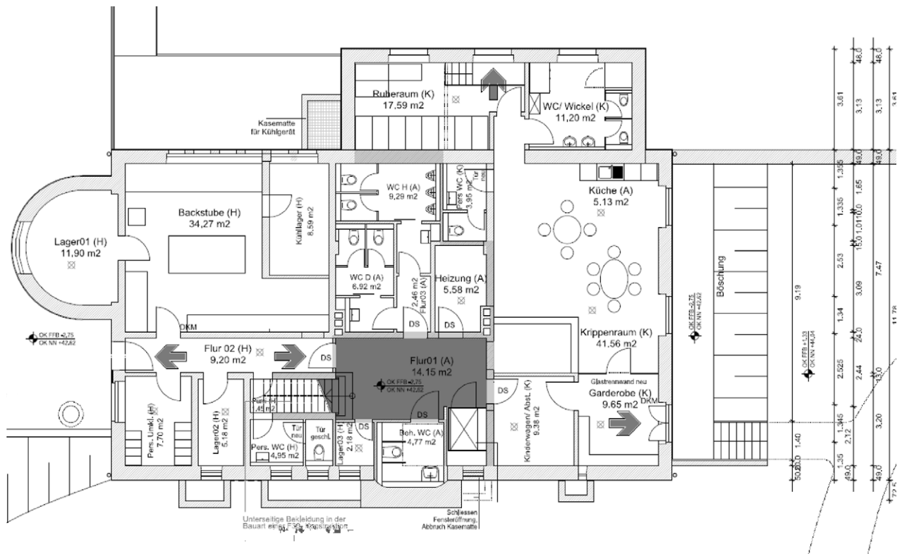
Fig. 2.3.7: Ohlendorff'sche Villa Basement
