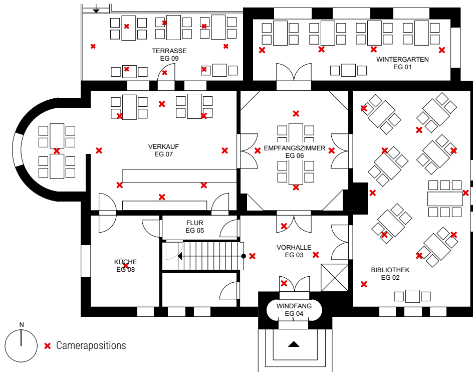
Fig. 2.5.2: Floorplan groundfloor
