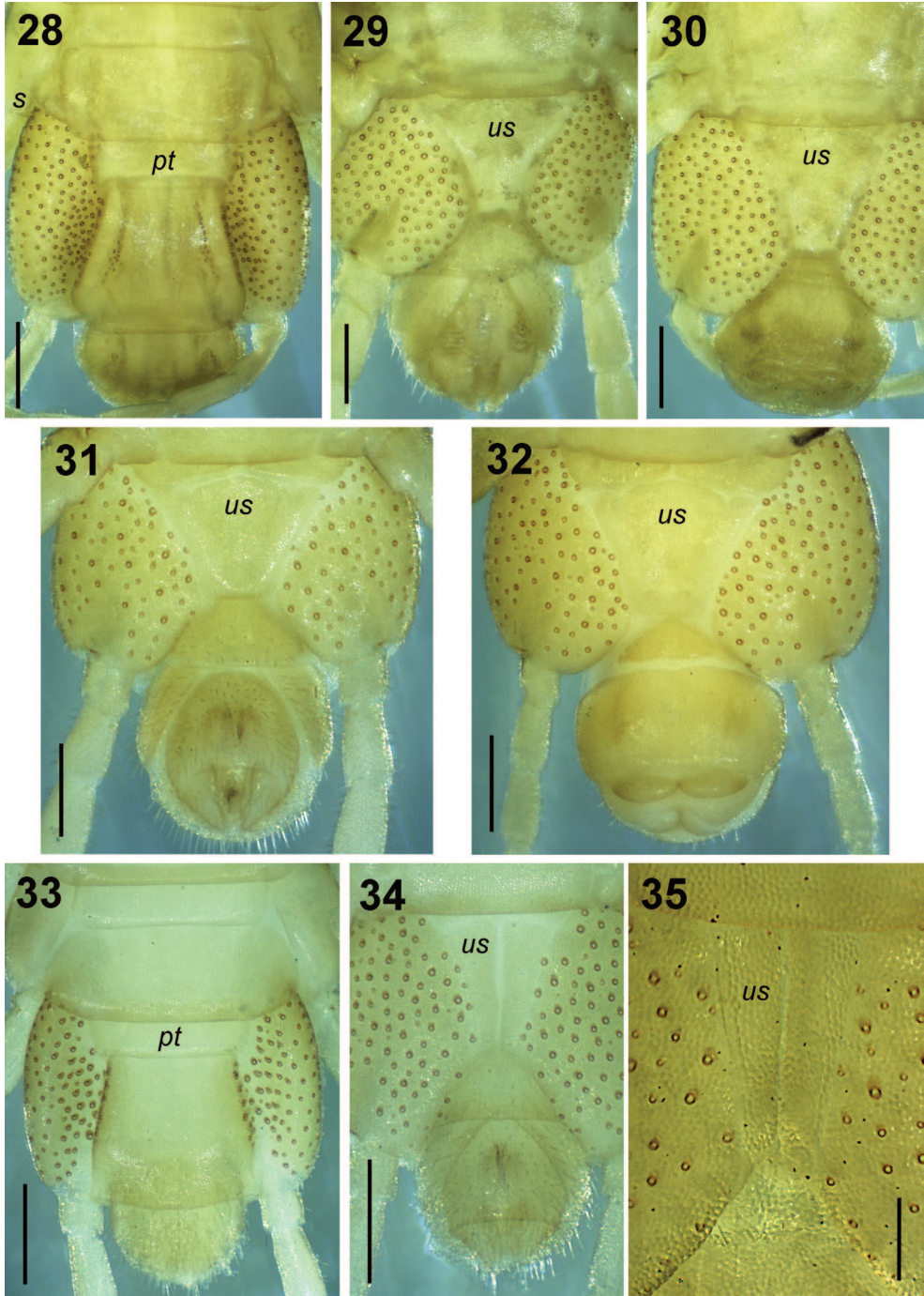
Fig. 28-35. – Stigmatogaster spp., derniers segments pédifères ( pt = prétergite du dernier segment pédifère ; s = pleurite stigmatifère du pénultième segment ; us = ultime sternite). – 28-32, S. dimidiata (Meinert) : 28, femelle syntype n°ZMUC 00020555, vue dorsale ; 29, mâle syntype, vue ventrale ; 30, femelle syntype, vue ventrale ; 31, mâle de Madrid, vue ventrale ; 32, femelle de Madrid. – 33-35, S. sardoa (Verhoeff) : 33-34, mâle de Ramatuelle (33, vue dorsale ; 34, vue ventrale) ; 35, femelle immature de Cavalaire-sur-Mer. Échelles : fig. 28-32 = 0,4 mm ; fig. 33-34 = 0,3 mm ; fig. 35 = 0,1 mm.
