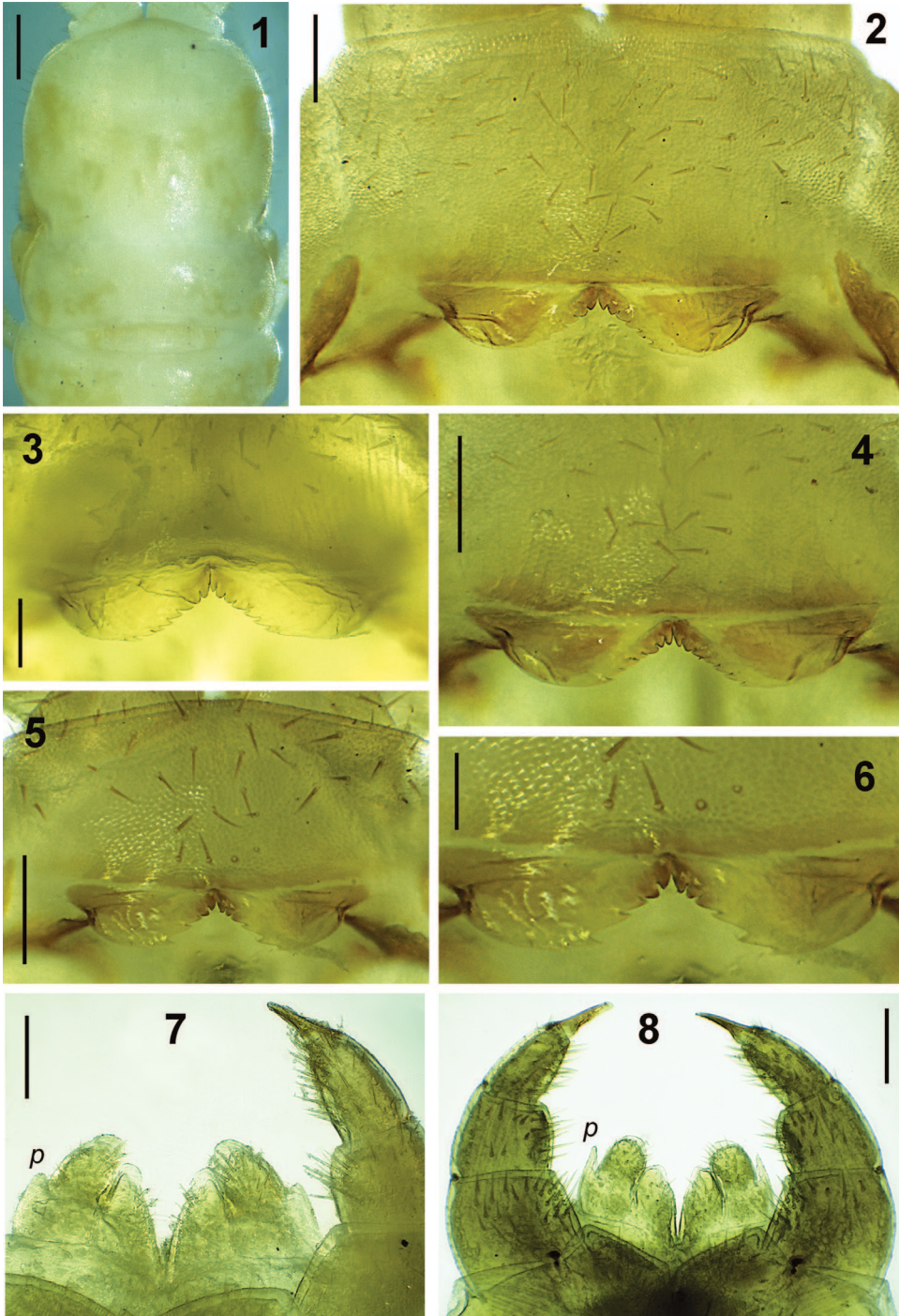
Fig. 1-8. – Stigmatogaster spp. – 1, S. sardoa , tête du mâle de Ramatuelle. – 2-6, Labre et clypeus : 2-4, S. dimidiata (Meinert) (2, femelle de Madrid; 3, mâle syntype n°ZMUC 00020555; 4, mâle de Madrid); 5-6, S. sardoa (5, mâle de Ramatuelle; 6, idem , zoom sur le labre). – 7-8, Maxilles ( p = palpe télodipital) : 7, S. sardoa (Verhoeff), femelle d’Ulassai; 8, S. dimidiata , mâle syntype n°ZMUC 00020555. Échelles : fig. 1 = 0,2 mm ; fig. 2-5, 7-8 = 0,1 mm ; fig. 6 = 0,05 mm.
