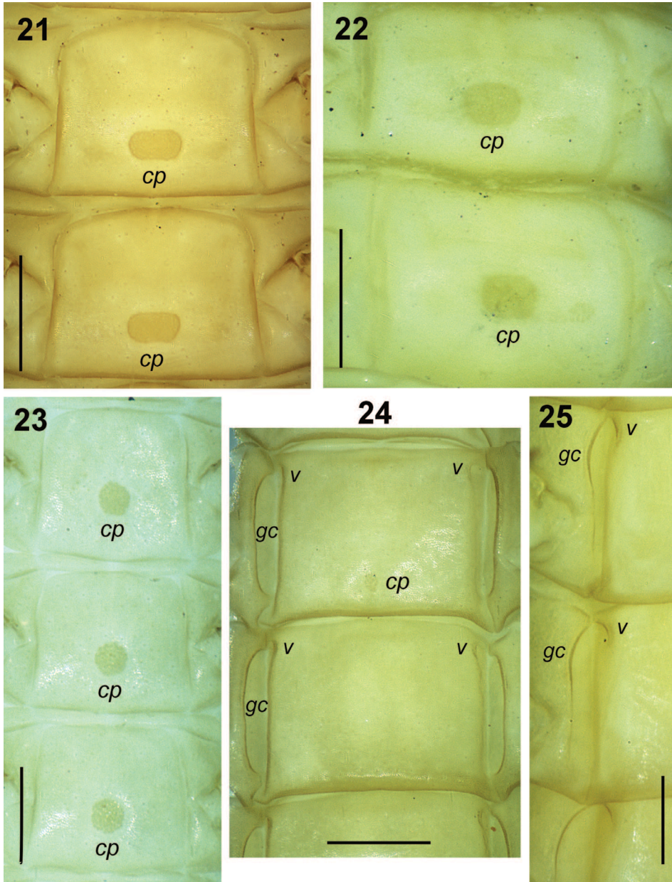
Fig. 21-25. – Stigmatogaster sardoa , segments pédifères, vue ventrale ( cp = champ poreux; v = fossette virgiforme; gc = gouttière coxale). – 21 , Femelle de Galtelli, segments 10-11. – 22 , Femelle d'Ulassai, segments 11-12. – 23-24 , Mâle de Ramatuelle : 23 , segments 23-26; 24 , segments 54-55. – 25 , Femelle d'Arbus, segments 59-60 (61), vue partielle. Échelles : fig. 21-22 = 0,5 mm; fig. 23-25 = 0,4 mm.
