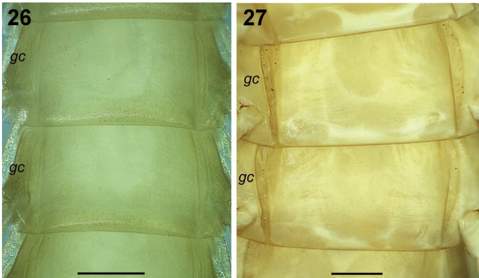
Fig. 26-27. – Stigmatogaster sardoa (Verhoeff), segments pédifères, vue ventrale (gc = gouttière coxale). – 26, Mâle de Ramatuelle, segments 111-112. – 27, Femelle de Galtelli, segments 118-119. Échelles = 0,3 mm.
