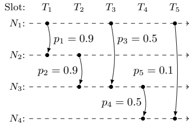
Fig. 7. Uncertain contact plan [23]
