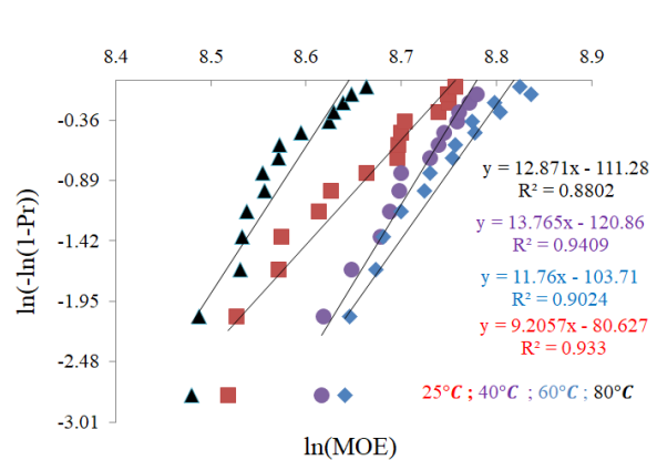
Fig. 2b : Détermination de m : Ayous.
