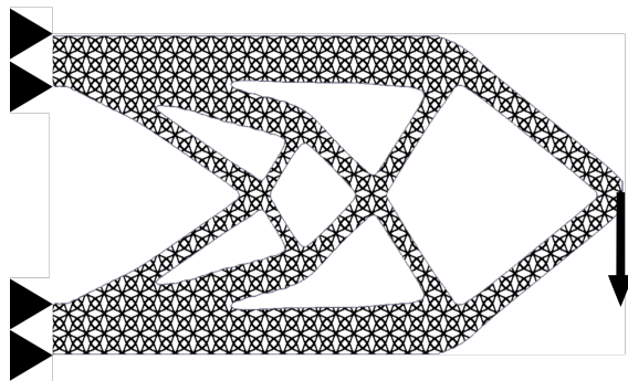
FIGURE 8 – Topologie optimisée du problème multi-échelle.
