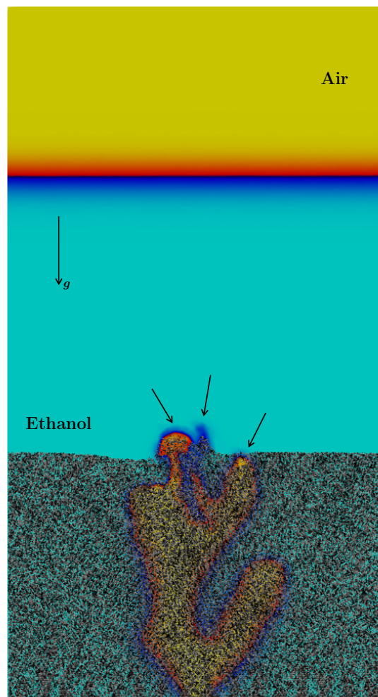
FIGURE 2 – Émission d'air à la surface du lit granulaire après 1.5 s
