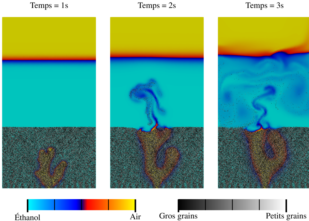
FIGURE 1 – Simulation bidimensionnelle de l'injection d'air, sous gravité, au sein d'une matrice granulaire immergée dans de l'éthanol. Le rayon moyen des grains de polystyrène vaut 0.495 \cdot 10^{-4} m, le diamètre d'injection est de 10^{-3} m et le débit d'injection vaut 0.2 L/min.
