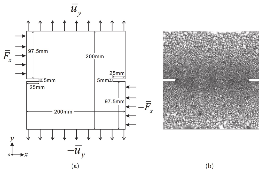
FIGURE 1 – La plaque bi-entaillée : (a) la géométrie et les conditions aux limites (b) le maillage pour l'exemple numérique
