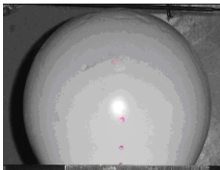
Figure 5 – Vue d'une bulle en ABS lors de soufflage
