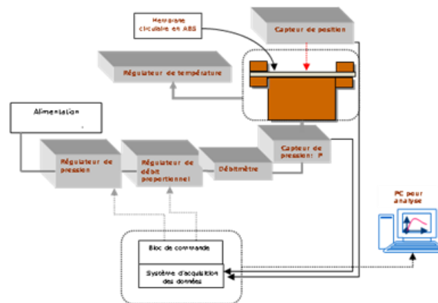
Figure 2 – Montage expérimental pour le soufflage
