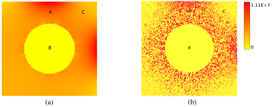
FIGURE 10 – Contrainte hydrostatique (Pa) par les deux approches (a) MEF (b) MED, où la valeur maximale de l'échelle des isovaleurs est celle calculée par la MEF
