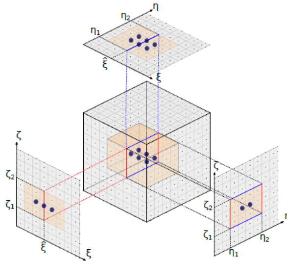
Figure 2 – Une mesh surface est définie par une valeur de knot spécifique \xi inséré et par une surface dans le plan des deux autres directions et bornée par [\eta_1, \eta_2] et [\zeta_1, \zeta_2] . La surface de coupe est projetée sur les plans (\xi, \eta) , (\eta, \zeta) et (\zeta, \xi) pour une meilleure visualisation.
