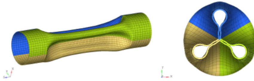
Figure 3 – Résultats de simulation pour le tube sous pression externe.
