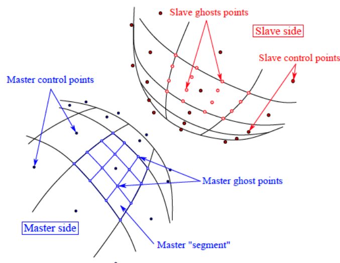
Figure 1 – Définition des surfaces maître et esclave pour deux géométries B-Spline quadratiques. La surface Spline et les points de contrôle sont tracés en noire. Le côté bleu représente le côté maître avec les segments construits à partir des points fictifs. Le côté rouge est le côté esclave avec les points fictifs associés.
