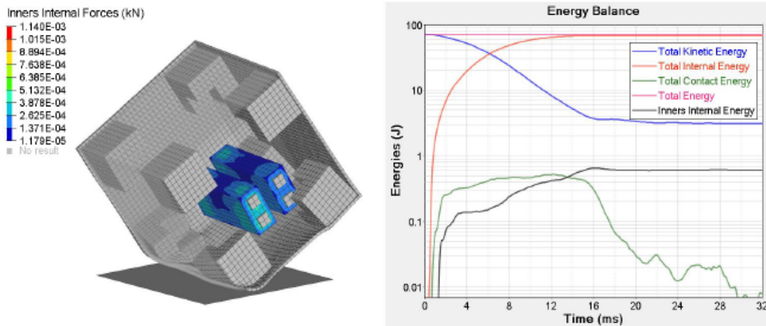
Figure 4 – Résultats de simulation de la chute du carton et bilan d'énergies.
