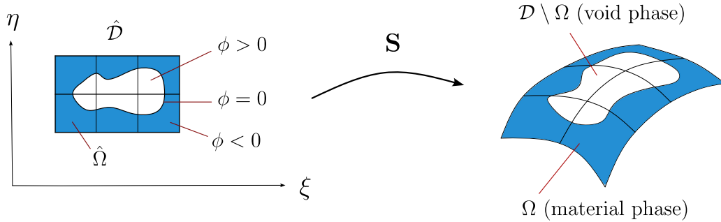
FIGURE 3 – Vue schématique de la méthode de surface de niveaux dans l'analyse isogéométrique. Une phase matérielle paramétrique \hat{\Omega}_k (en bleu) est définie comme l'ensemble de points dans l'espace paramétrique où la fonction de surface de niveaux \phi_k est négative. L'image de \hat{\Omega}_k par la surface NURBS \mathbf{S}_k définit la forme \Omega_k (en bleu) en tant que sous-ensemble de la surface médiane de la coque. L'ensemble \mathcal{D}_k \setminus \Omega_k ayant des propriétés matérielles faibles est appelé la phase vide et il agit comme une région vide.
