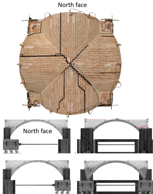
FIGURE 6 – Sera : faciès de rupture
