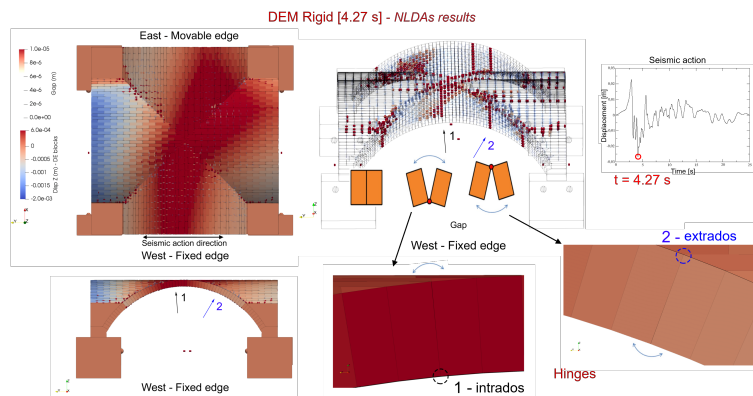
FIGURE 7 – Sera : résultats numériques
