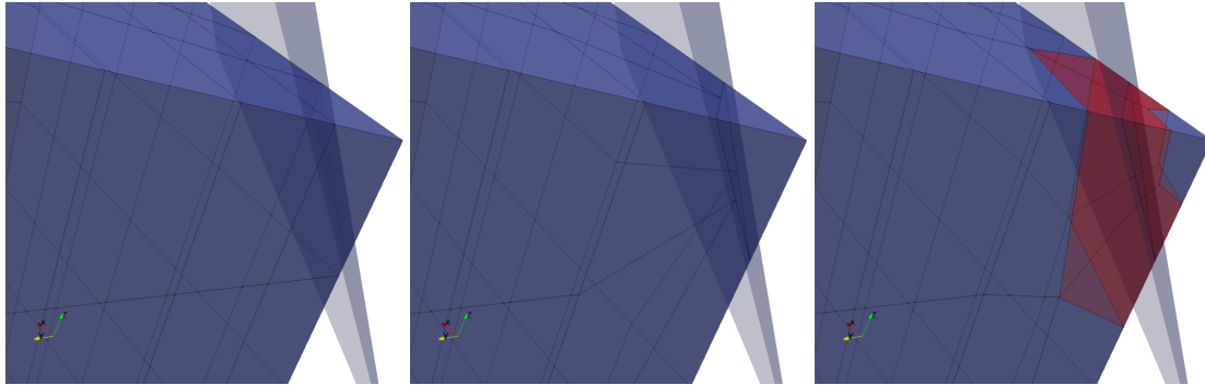
FIGURE 3 – La region opaque grise est la surface divisée, la region opaque bleue représente le maillage. Le maillage d'origine est à gauche, le maillage avec l'algorithme Smart Octree au milieu, et le maillage "pillowing" à droite. On peut remarquer la présence des doublets au milieu. Les éléments rouges ont été générés lors du processus de "pillowing".
