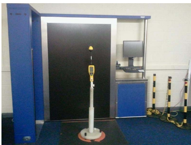
Figure 3 : Photographie de l'appareil de mesures de champs électromagnétiques (laboratoire CEI)
