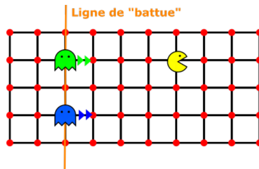
FIGURE 13 – Illustration de la stratégie en battue. Les fantômes se mettent en colonnes et forment une ligne de « battue » infranchissable par Pac-Man. Ils peuvent ensuite acculer Pac-Man sur le bord.
