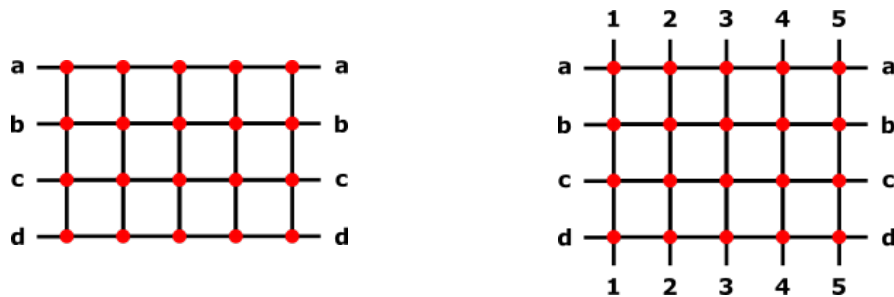
FIGURE 12 – Un exemple de bande (à gauche) et de tore (à droite). Chaque demie-arrête du bord doit être reliée à la demie-arrête à l'opposé avec la même lettre ou le même numéro.
