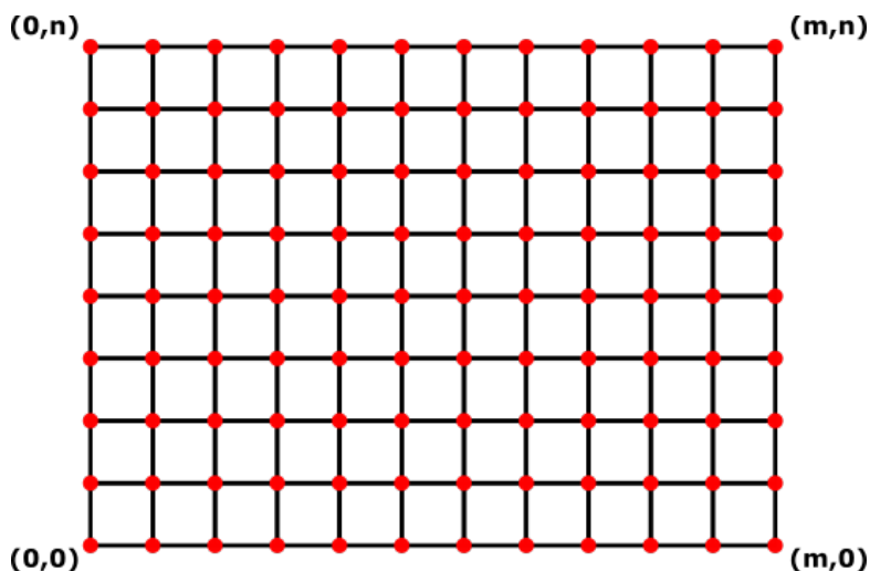
FIGURE 1 – Exemple de grille avec m = 11 et n = 8 .
