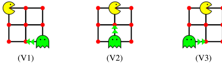
FIGURE 3 – Illustrations des déplacements pour le fantôme vert.
