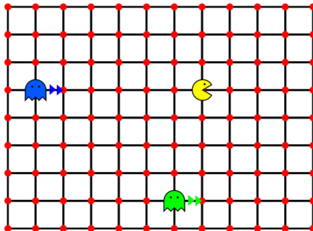
FIGURE 8 – Exemple 4 de coup du joueur F . Ici Pac-Man s’est déplacé vers la droite ce qui a brisé l’alignement avec le fantôme vert. Ce dernier rectifie donc l’alignement tandis que le fantôme bleu, bien aligné, se rapproche.
