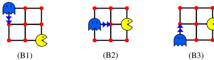
FIGURE 4 – Illustrations des déplacements pour le fantôme bleu.
