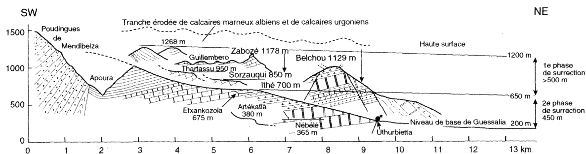
Figure 2 : Représentation schématique des niveaux fluvio-karstiques et endokarstiques étagés et correspondance avec les phases de surrection plio-quadernaire.
