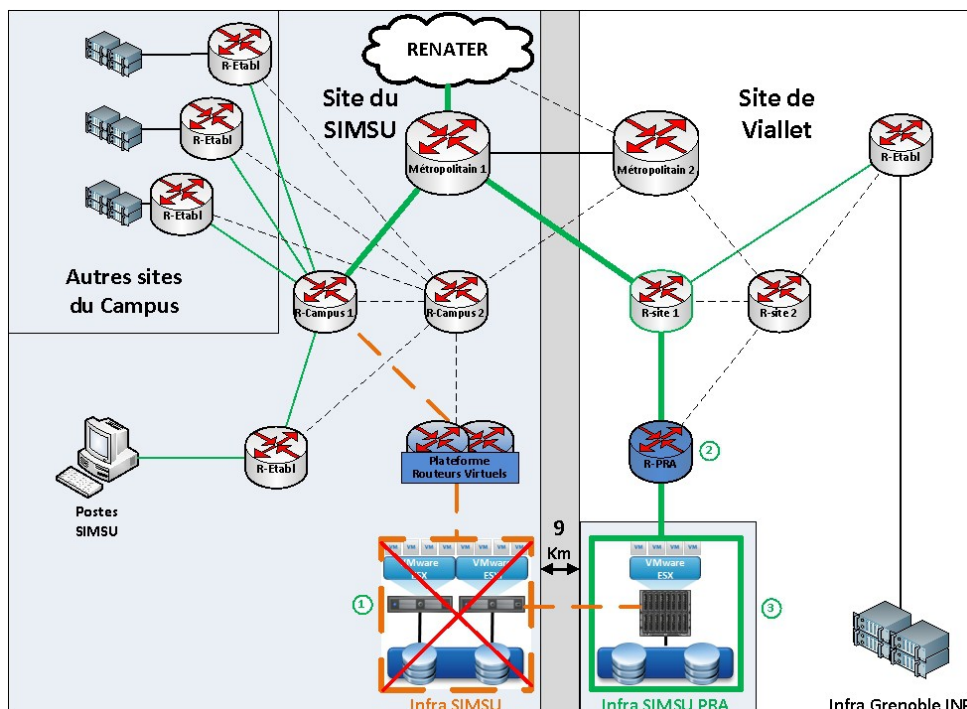
Figure 3-Bascule réseau
