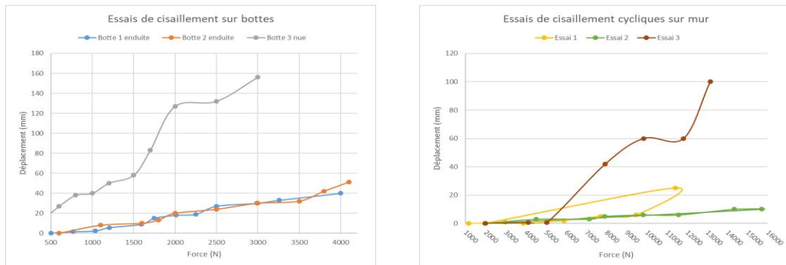
Figure 3 Graphes des essais de cisaillement sur bottes et sur mur (IUT de Nîmes, 2019)
