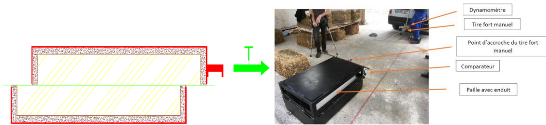
Figure 2 Principe de l'essai de cisaillement sur bottes (IUT de Nîmes, 2019)
