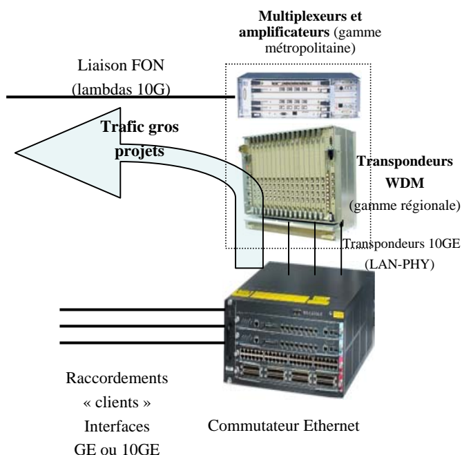
Figure 4 – Nœud RENATER-4 DWDM
