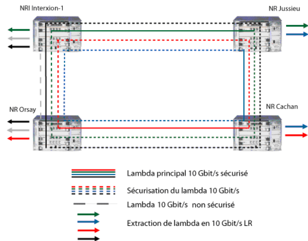
Figure 1 – DWDM en Île-de-France
