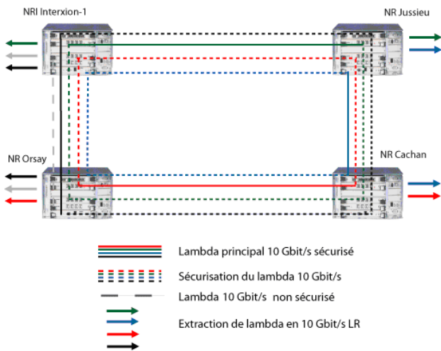
Figure 1 – DWDM en Île-de-France
