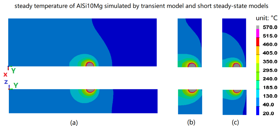
FIGURE 6 – Température stationnaire de l'AlSi10Mg : (a) modèle transitoire, (b) modèle court stationnaire avec conditions aux limites classiques, (c) modèle court stationnaire avec conditions aux limites proposées.
