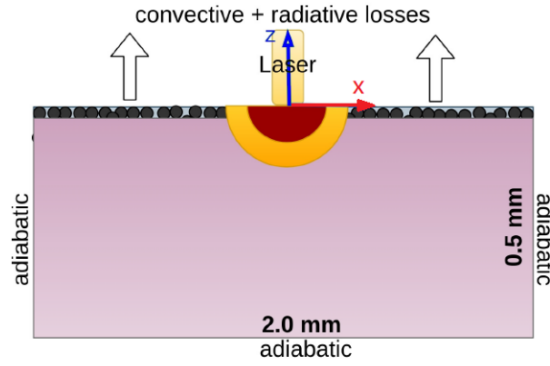
FIGURE 3 – Modèle et conditions aux limites thermique : section transversale.
