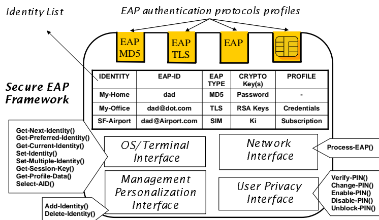
Figure 9– Architecture globale d'une carte EAP.
