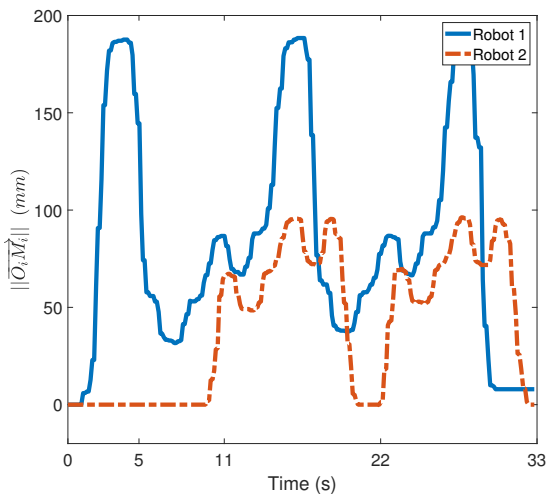
Figure 7: (Sc3) Robot 1 : \|\overrightarrow{O_1M_1}\| ; Robot 2 : \|\overrightarrow{O_2M_2}\|
