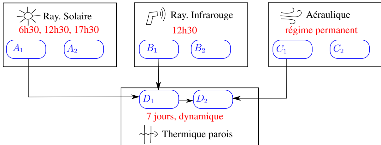
Figure 2 : Huit configurations étudiées ( A_1, A_2, B_1, B_2, C_1, C_2, D_1, D_2 ) pour l'analyse du rayonnement solaire et infrarouge, de l'aérodynamique et de la thermique du solide. Les heures sont données en UTC et correspondent au 18/07/2022.
