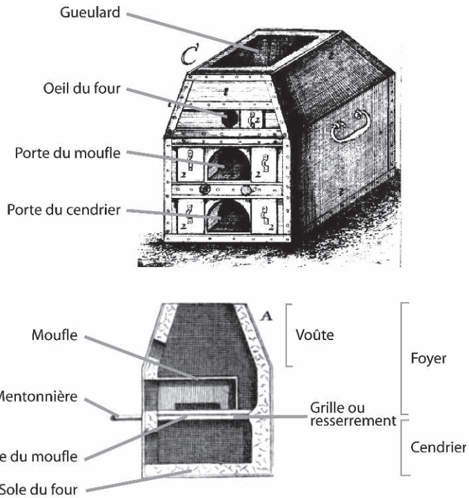
Fig. 1. - Schéma du four à moufle
