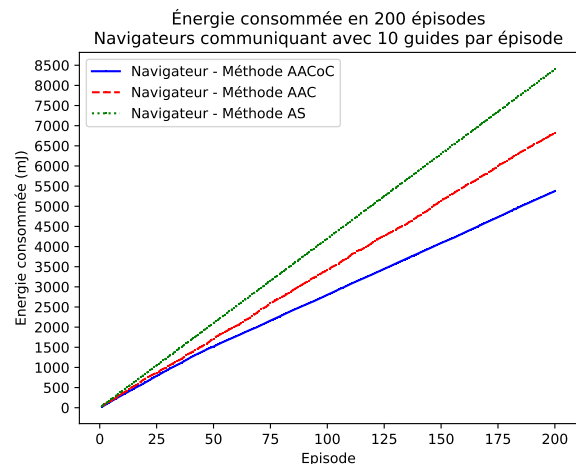
FIGURE 3 – Énergie consommée pour l’authentification en 200 épisodes
