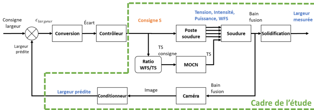
Figure 1 : Framework de l'asservissement et cadre de l'étude. En vert : le cadre de l'étude. En orange : la consigne. En bleu : les différentes grandeurs physiques mesurées.
