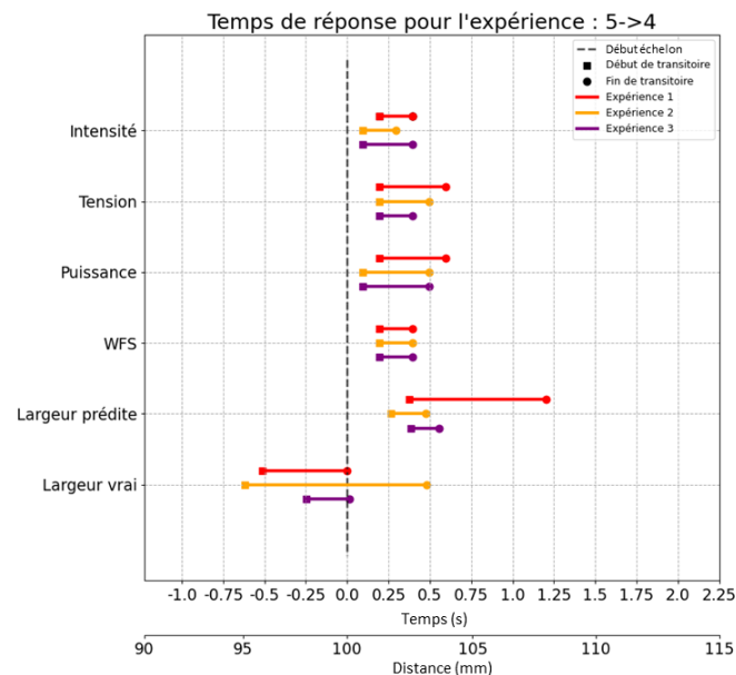
Figure 7 : Temps et distance de réponse pour un échelon de S = 5 à S = 4
