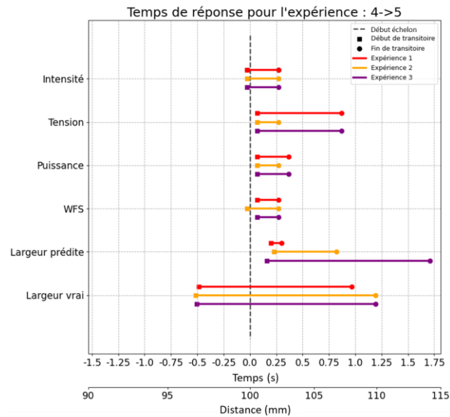
Figure 6 : Temps et distance de réponse pour un échelon de S = 4 à S = 5
