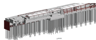
(d) Concrete layout showing steel piles
