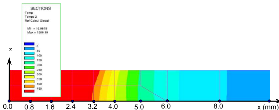
Figure 11. Distribution transversale des températures au temps t = 2s
