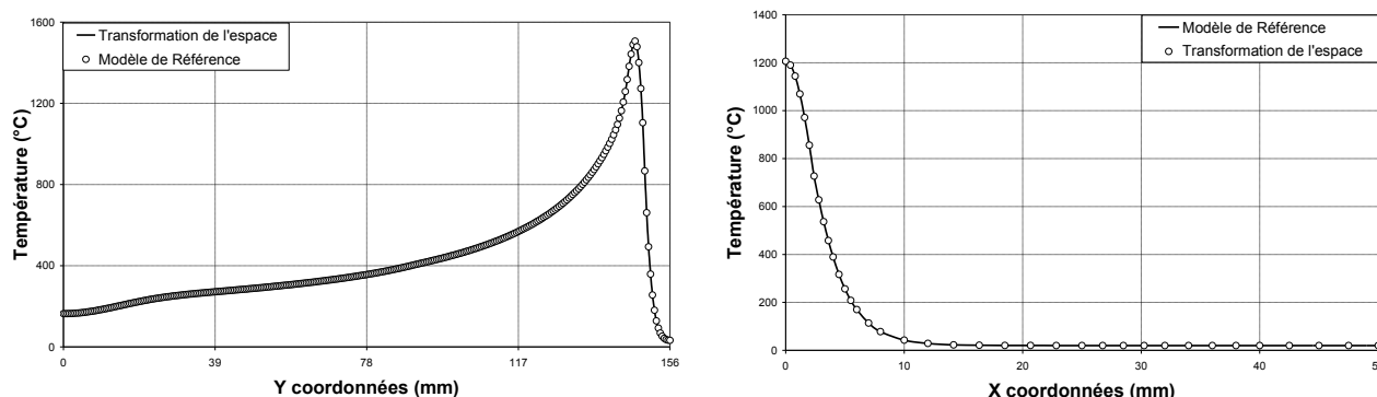
Figure 10. Distribution des températures au temps t = 7,2 s A gauche : ligne 1 ( x = 0 mm ) ; à droite : ligne 2 ( y = 144 mm )
