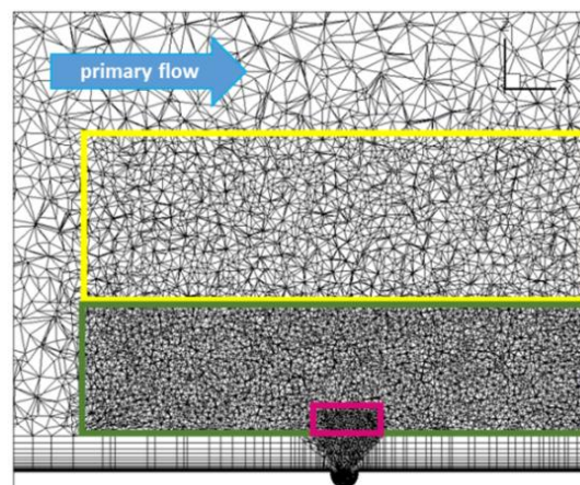
Figure 4 – Vue générale du maillage côté écoulement primaire
