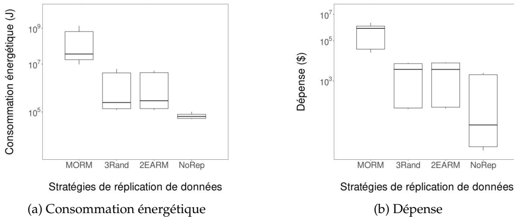
FIGURE 1 – Résultats des fonctions objectifs
