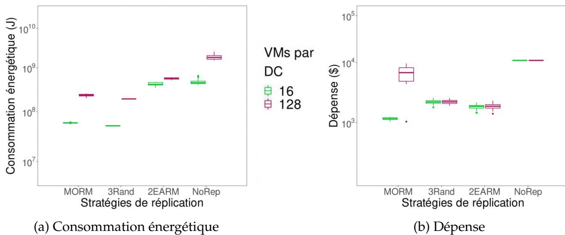
FIGURE 2 – Résultats des exécutions
