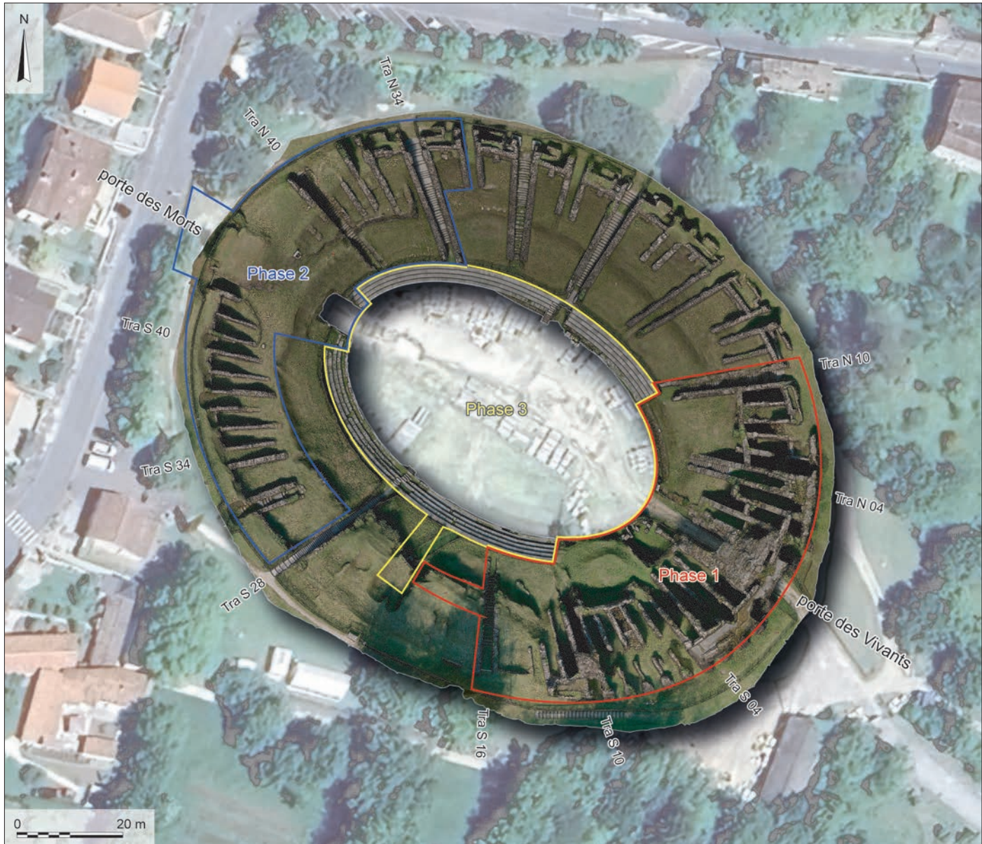
Fig. 1 – Localisation des secteurs d'intervention sur le site de l'amphithéâtre de Saintes (Charente-Maritime), phases 1 à 3 (DAO: C. Gay, SAD17; sur fond Google satellite, Aerial Data).
