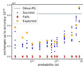
Fig. 2. madelon dataset
