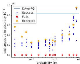
Fig. 2. madelon dataset
