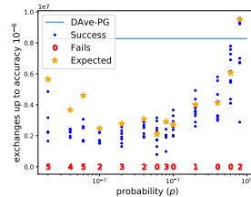
Fig. 2. madelon dataset
