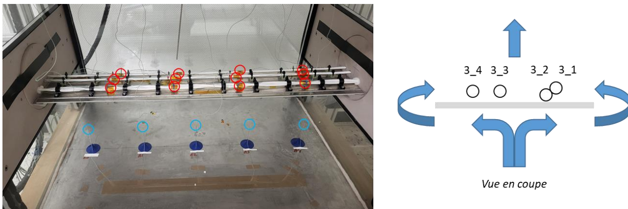
Figure 4 : Configuration 3 et schéma des câbles sur la plaque aluminium
