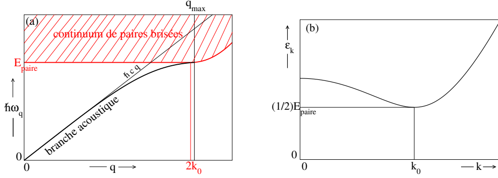
FIGURE 5. Énergie de différents types d'excitations d'un gaz homogène non polarisé de fermions à deux composantes à température nulle, en fonction de leur nombre d'onde q ou k . (a) Branche d'excitation acoustique \hbar\omega_{\mathbf{q}} de départ linéaire \hbar c q ( c est la vitesse du son), limitée supérieurement par le continuum de paire brisée (zone hachurée) dont elle vient ici tangenter le bord inférieur en le point terminal de nombre d'onde q_{\max} . Sous l'effet d'une excitation percussionnelle de vecteur d'onde \mathbf{q} , une paire liée \uparrow\downarrow du condensat de paires, initialement au repos, se dissocie en deux quasi-particules fermionique \gamma de spins opposés (voir texte), de vecteurs d'onde \mathbf{k} et \mathbf{k}' = \mathbf{q} - \mathbf{k} et d'énergies \varepsilon_{\mathbf{k}} et \varepsilon_{\mathbf{k}'} ; comme le vecteur \mathbf{k} n'est pas contraint (pas de conservation de l'énergie), il apparaît un continuum d'énergies finales \{\varepsilon_{\mathbf{k}} + \varepsilon_{\mathbf{q}-\mathbf{k}}, \mathbf{k} \in \mathbb{R}^3\} . Pour la force des interactions choisie sur la figure ( |\Delta|/\mu = 0,84 soit 1/k_{\text{F}}a \approx -0,16 d'après la théorie BCS, avec \mu le potentiel chimique du gaz et \Delta le paramètre d'ordre complexe du condensat de paires), la branche acoustique est de départ concave ( \gamma < 0 dans l'équation (33)) et (b) la relation de dispersion \varepsilon_{\mathbf{k}} présente un minimum E_{\text{paire}}/2 en k = k_0 > 0 ; le bord inférieur du continuum vaut donc exactement E_{\text{paire}} , du moins tant qu'on peut avoir k = k' = k_0 donc tant que q = |\mathbf{k} + \mathbf{k}'| \leq 2k_0 . Les relations de dispersion représentées, approchées, sont celles de la théorie BCS pour \varepsilon_{\mathbf{k}} et de la RPA d'Anderson pour \hbar\omega_{\mathbf{q}} . Selon la force des interactions, le domaine d'existence en q de la branche acoustique peut également être non compact, connexe q \in ]0, +\infty[ ou pas q \in ]0, q_{\max}[ \cup ]q_{\min}, +\infty[ ( q_{\min} > q_{\max} ) [42]; la concavité de la branche est elle aussi variable [43]; enfin, k_0 = 0 et E_{\text{paire}} = 2(\mu^2 + |\Delta|^2)^{1/2} si \mu < 0 , k_0 = (2m\mu)^{1/2}/\hbar et E_{\text{paire}} = 2|\Delta| sinon.
