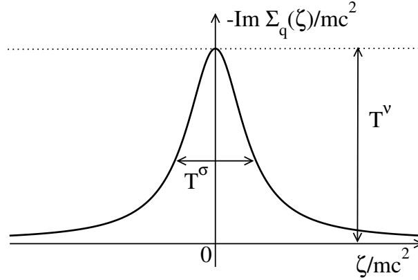
FIGURE 8. Dans la limite T \rightarrow 0 , on admet que l'ordre de grandeur et la largeur typique de la fonction \text{Im}\Sigma_{\mathbf{q}}(\zeta) près de \zeta = i0^+ sont caractérisés par deux lois de puissance en température, d'exposants \nu et \sigma .
