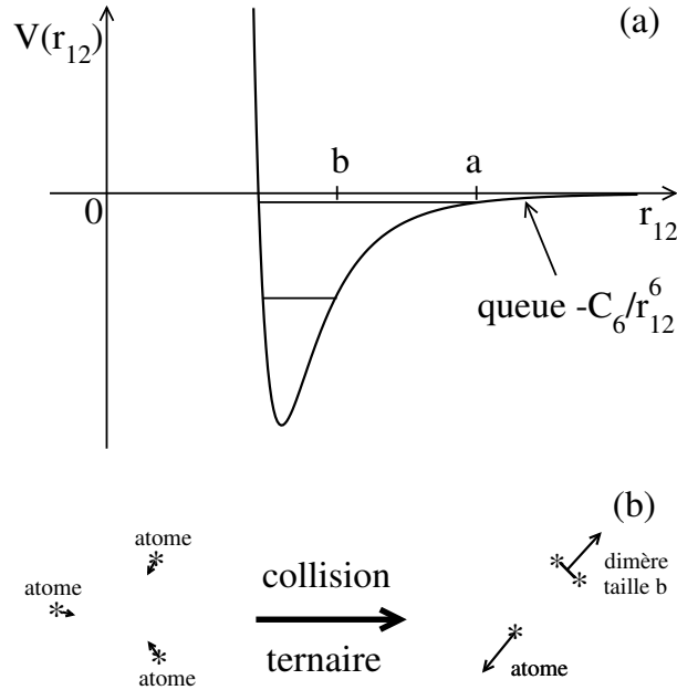
FIGURE 1. (a) Représentation schématique de l’interaction de van der Waals résonnante ( |a| \gg b ) entre les fermions \uparrow et \downarrow . Le potentiel admet au moins un état fortement lié d’extension de l’ordre de la longueur de van der Waals b \simeq (mC_6/\hbar^2) donc d’énergie de liaison \simeq \hbar^2/mb^2 et, dans le cas d’une longueur de diffusion a > 0 comme sur la figure, un dernier niveau d’énergie d’extension a (d’énergie de liaison \hbar^2/ma^2 ) sur « le point de disparaître »; si a était grande mais négative ( |a| \gg b, a < 0 ), cet état faiblement lié serait sur « le point d’apparaître ». (b) L’état dimère fortement lié peut être peuplé par des collisions à trois corps et est à l’origine de pertes de particules dans le gaz de fermions, dites pertes à trois corps. Les flèches représentent les quantités de mouvement avant et après la collision.
