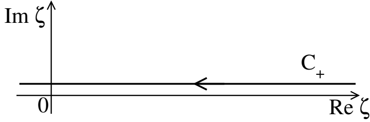
FIGURE 7. Chemin d'intégration dans le plan complexe suivi par l'équation (47).
