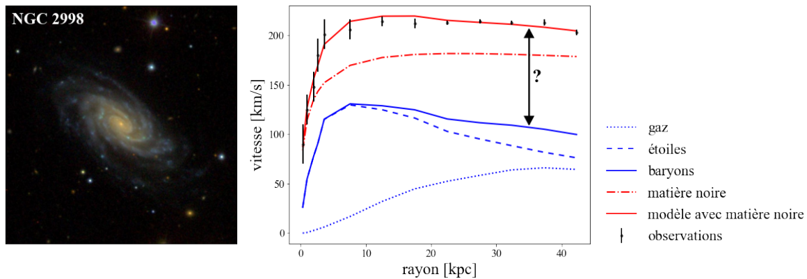
Figure 3. La courbe de rotation observée de la galaxie spirale NGC 2998 peut être expliquée en ajoutant les contributions du gaz, des étoiles, et d'un halo sphérique de matière noire. La matière visible, dite « baryonique », qui comprend le gaz et les étoiles, ne permet pas à elle seule de rendre compte des vitesses de rotation mesurées. La modification de la gravitation de Milgrom peut, quant à elle, rendre compte de cette observation sans matière noire. Crédits : SDSS pour l'image de la galaxie, Lelli et al. (2016) pour la courbe de rotation observée 41 .
