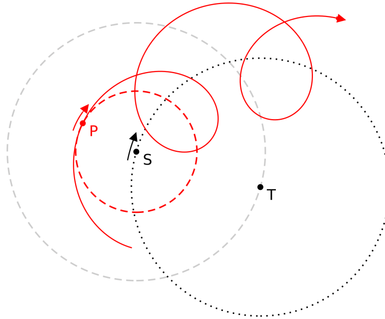
Figure 1. Dans le modèle géocentrique de Ptolémée, le mouvement d'une planète (P) par rapport à la Terre (T) est décrit par un épicycle dont le centre (S) suit une trajectoire circulaire autour de la Terre le long du cercle déférent. La courbe rouge indique le mouvement de la planète par rapport à la Terre, le cercle pointillé rouge l'épicycle, et le cercle pointillé noir le cercle déférent. Cette situation pourrait toutefois tout aussi bien être décrite en supposant que la Terre et la planète orbitent toutes deux autour de S, comme indiqué par le cercle pointillé gris.
