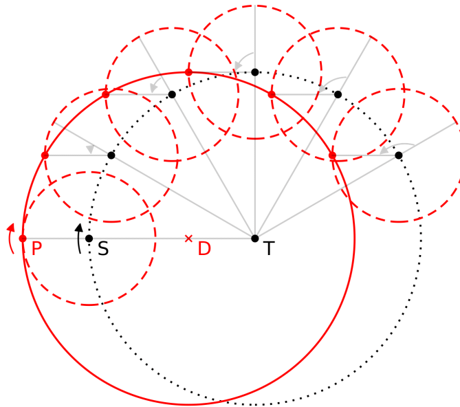
Figure 2. La trajectoire d'une planète (P) décrite par cercle excentrique (cercle rouge, de centre D) peut tout aussi bien être décrite par un épicycle (cercle rouge pointillé, de centre S en rotation autour de T) dont la période orbitale est égale à celle de son centre.
