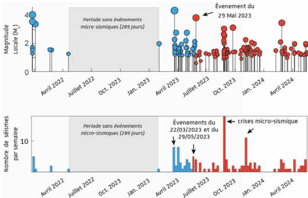
Figure 1-3 Sismicité dans un rayon de 5 km autour de l'épicentre du séisme du 29 mai 2023 enregistrée par le BCSF-Rénaiss entre janvier 2022 et mai 2024. B. Derode, EOST-ITES, mai 2024.
