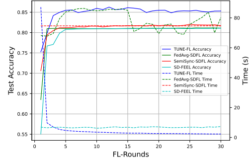
(a) UNSW-NB15
