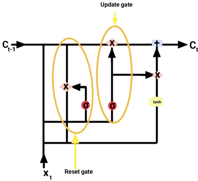
Fig. 1. RNN-GRU Schema
