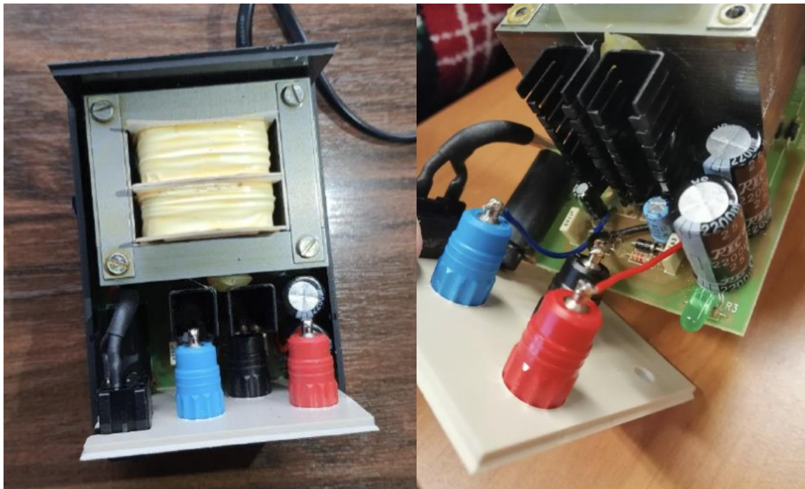
Figure 11 Photos de l'alimentation réparée
