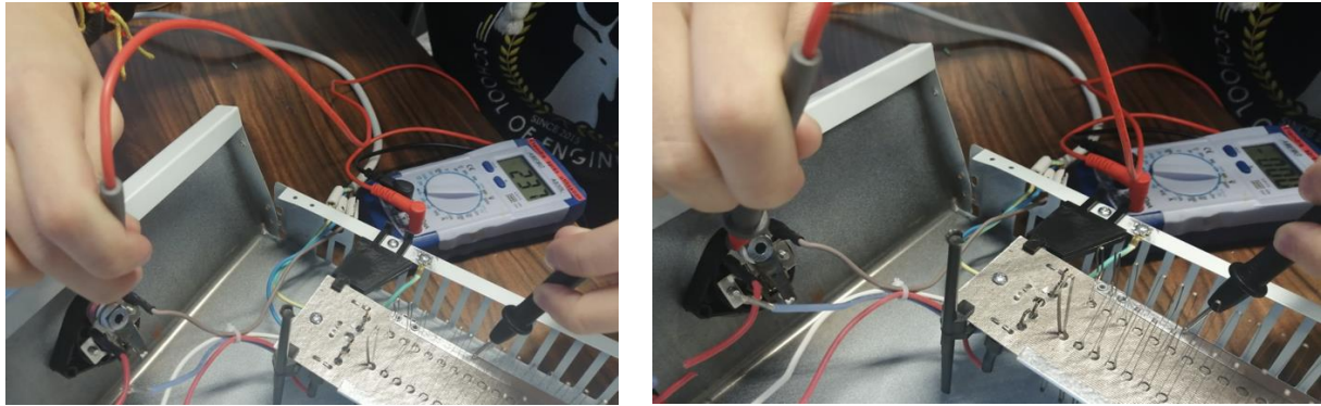
Figure 7 Photos prises lors du diagnostic : on mesure la tension entre différents points
