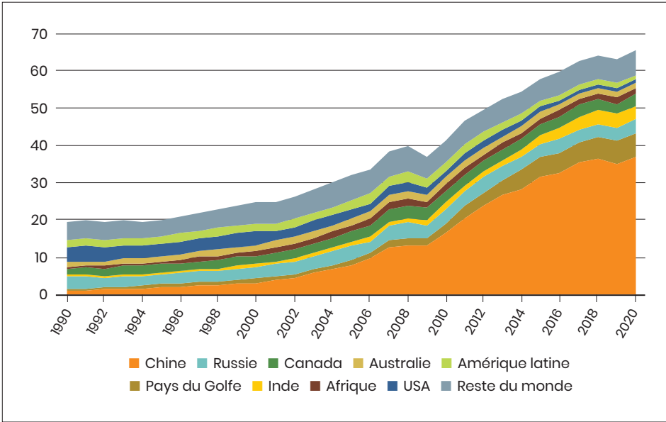
Graphique 9. Production mondiale d'aluminium (million de tonnes)
