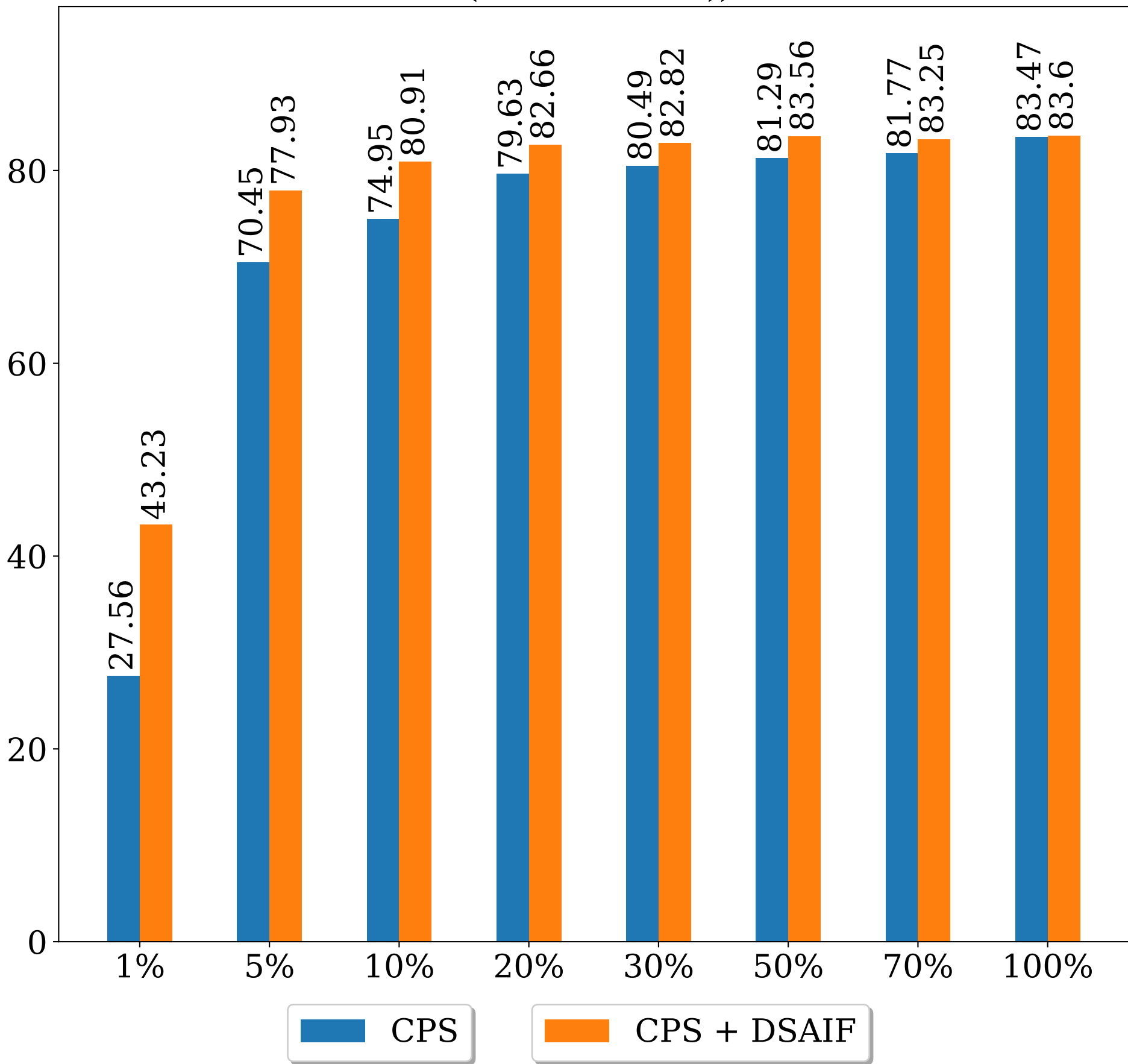
Dice Coefficient (%) (Pancreas-NIH)
