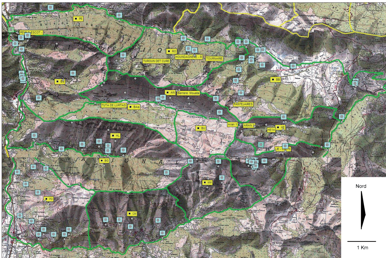
Figure 3 - Carte topographique et localisation des 145 grottes et gouffres et des 76 sources (extraits des cartes IGN Oloron-Sainte-Marie - vallée d'Aspe n° 1546 OT et Laruns - Gourette - Aubisque - vallée d'Ossau n° 1546 ET, © IGN - Paris 2009 - Autorisation n° 2200952 ; base de données du Comité Départemental de Spéléologie 64 ; synthèse F. Ichas).
