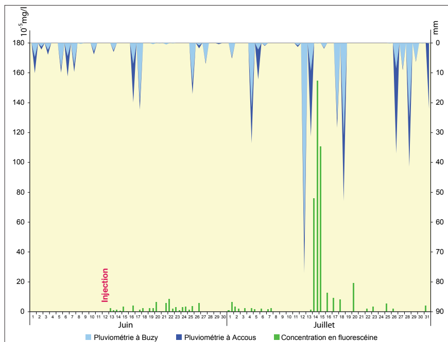
Figure 5 - Traçage à l'uranine dans le gouffre du Col d'Aran n° 1 le 12 juin 1999. La station météorologique de Buzy est située à 11 km au nord-nord-est du col d'Aran et la station d'Accous à 10,5 km au sud-ouest (données météorologiques : Météo France)
