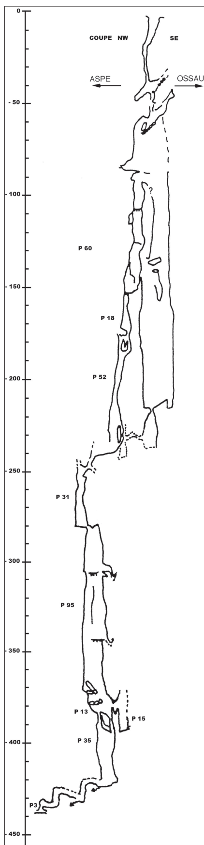
Figure 4 - Coupe du gouffre d'Aran n° 1. Topographie : P.-A. Acquier, J.-P. Besson, G. Cazenave, P. Fillon, C. et J. Labat, A. Levêque. Section of Aran n° 1 cave.
