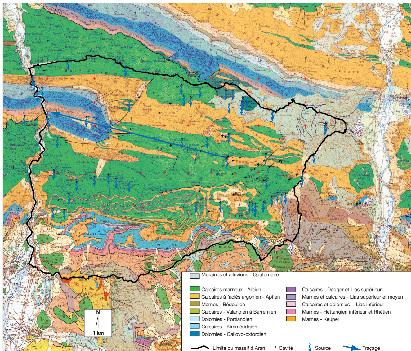
Figure 2 - Carte hydrogéologique d'Aran. Le massif totalise une superficie d'environ 75 km 2 . Les entrées de cavités se localisent de façon préférentielle dans les calcaires urgo-aptiens ; les sources sont situées sur les calcaires marneux albiens (extraits de la carte géologique de la France au 1/50 000e, feuilles Oloron-Sainte-Marie n° 1051 et Laruns-Somport n° 1069 - © BRGM - www.brgm.fr - Autorisation R09/30 Ed. ; base de données du Comité Départemental de Spéléologie 64).
